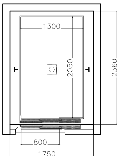
HIDRAULICO EMPUJE CENTRAL.
