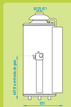
VISTA FRENTE
